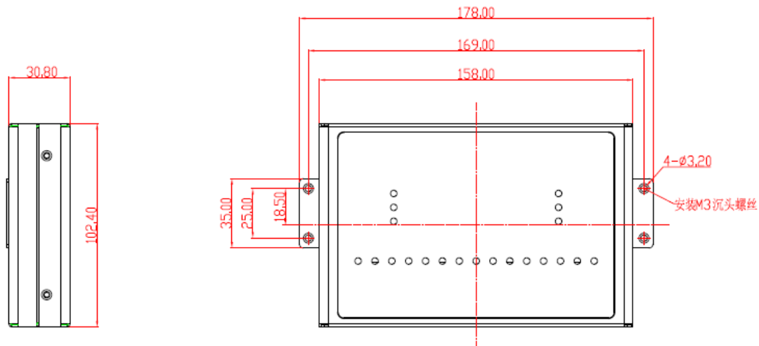
图 1.1 机械尺寸
